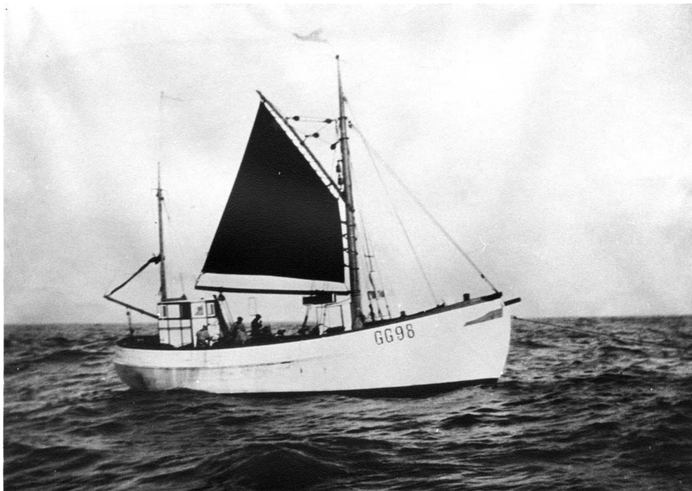
GG 98 VERONA TÅNGEN Byggd på Karlstad varv 1928. Här under snurrevadsfiske Br.ton 44,6 L 16,18 B 5,77 D 2,65 m. Motor June Munktell 1-cyl. 50 hk.
