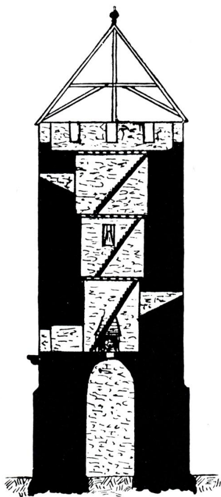
Den enkla borgen, som inte var avsedd till permanent bostad, var i regel ett fristående runt eller kvadratisk torn av ungefär 27 meters höjd och 9,5 meters sida. Tvärsnitt efter Piper.
