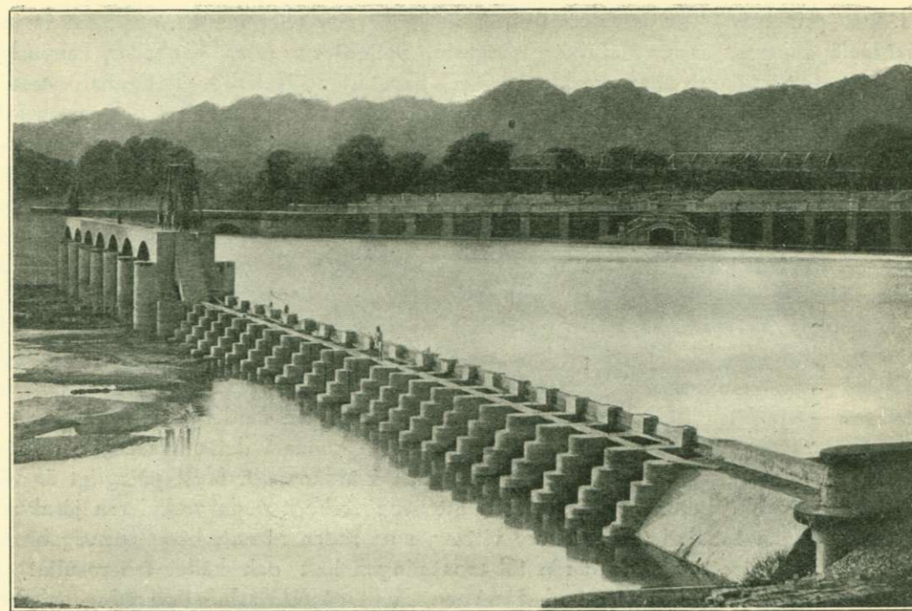
Dammanläggning i Gangeskanalen (Indien).
