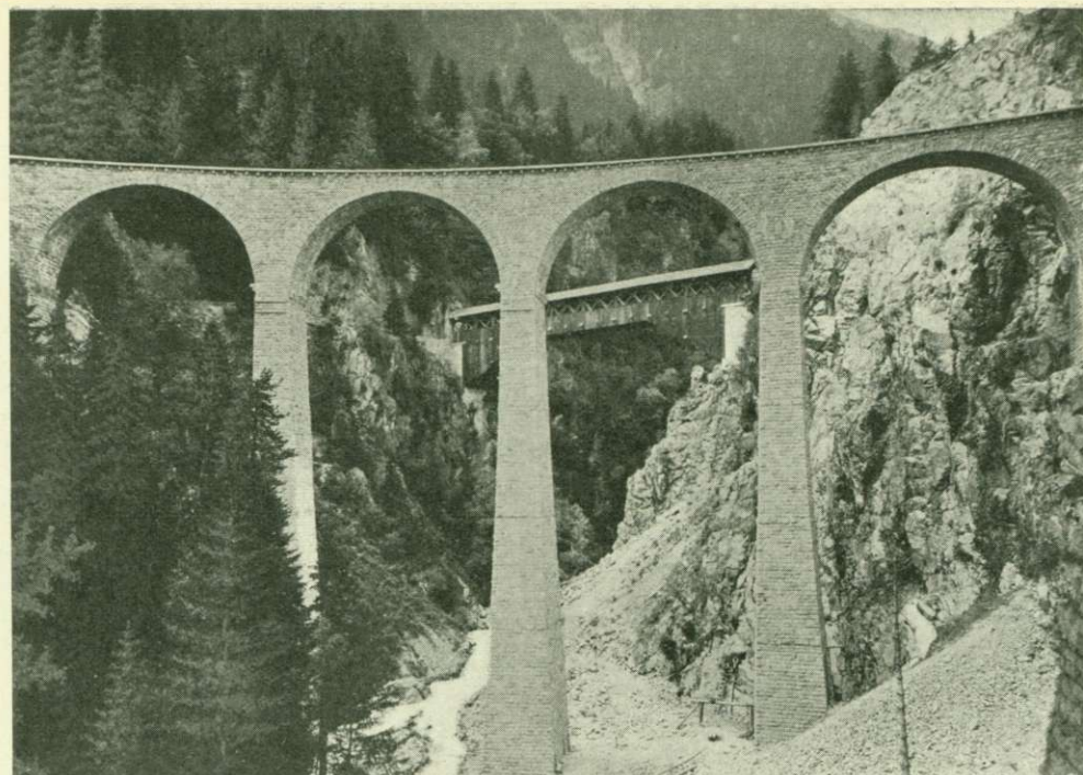
Järnvägsbro på Albulabanan (Kantonen Graubünden).
