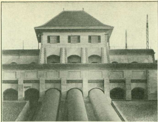
Kraftstationen vid Kallnach, kantonen Bern. Det s. k. intaget. Kraftiga men goda former i byggnaden.
