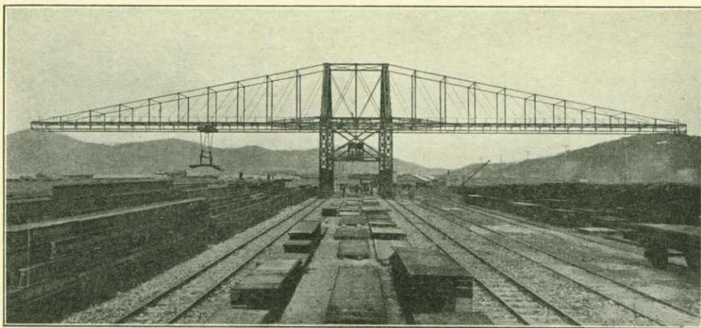
Kran för kaiserliga japanska stålverken.
