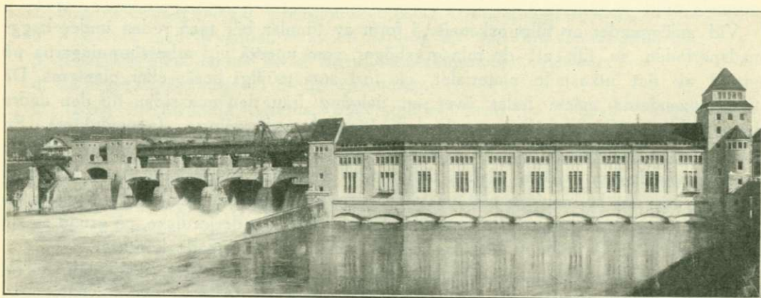
Kraftstationen vid Laufen, kantonen Zürich. Dammanläggning med turbinhus av monumental verkan.
