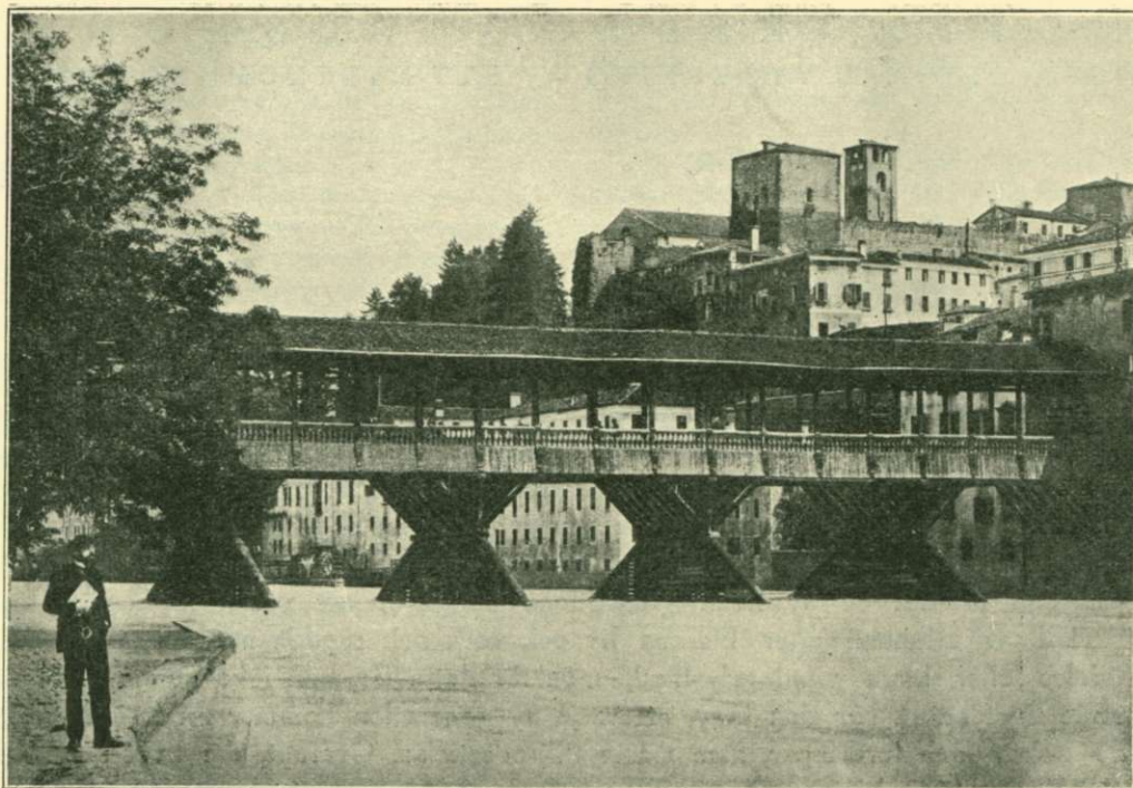
Gammal träbro över Brenta vid Bassano (Italien).
