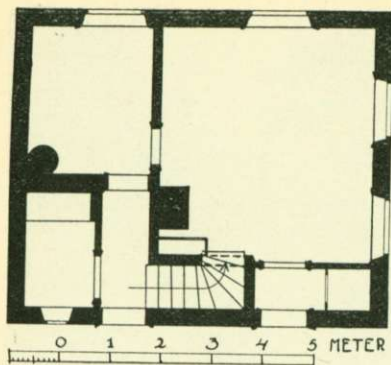
Ett av småhusen Fjällgatan 30. Plan av bottenvåningen.
