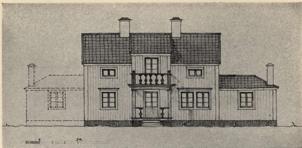
2. Fasadritning till hus i Motala.
