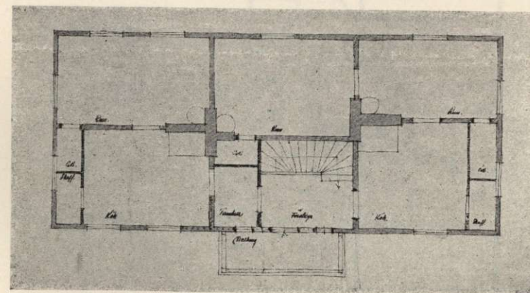
3—5. Ombyggnad av gammal gård i Järbo, Hälsingland.
