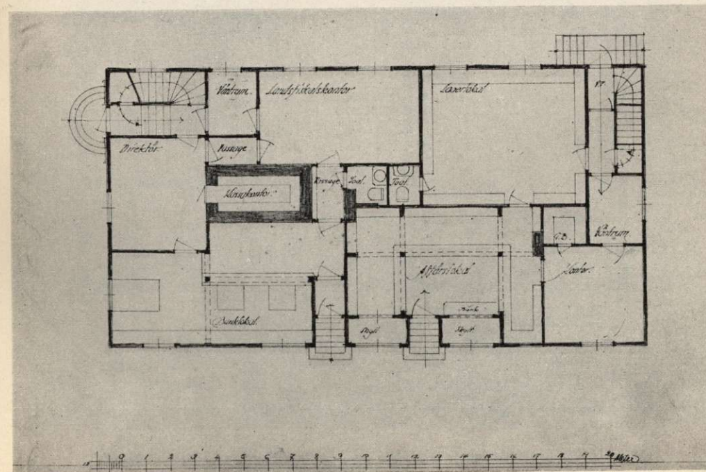
8—9. Ritning till affärshus i stationssamhälle i Dalarna,
