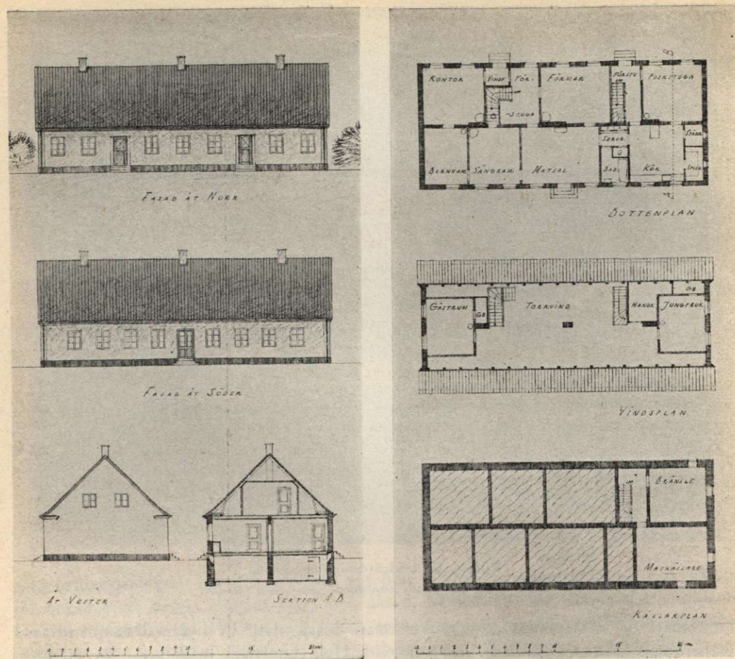
Ritning till boningslänga vid skänst jordbruk, utförd av elev vid Hvilans folshögskola, vinterkursen 1923—24.
