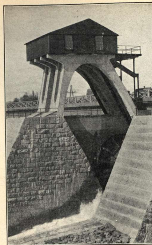
Från Forshuvudforsens kraftverk.
