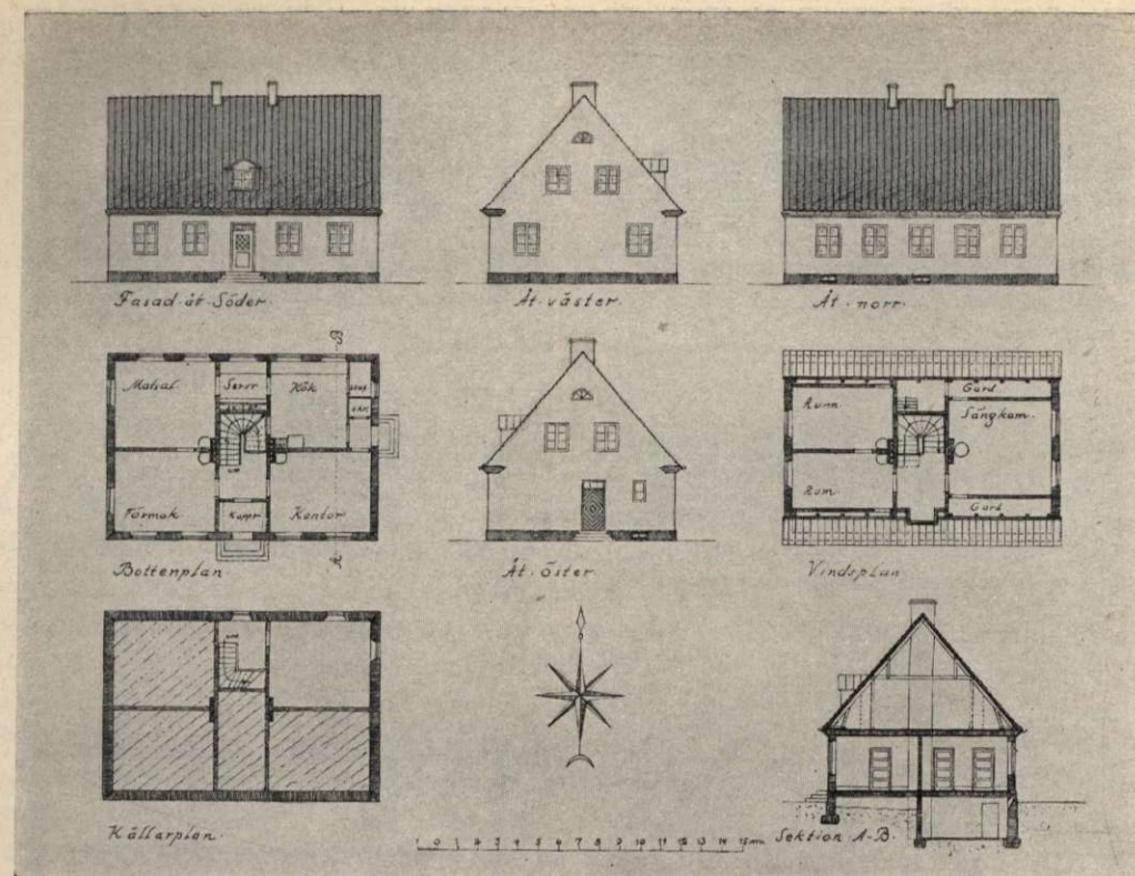
Ritning till trädgårdsmästarebostad, utförd av elev vid Hvilans folkhögskola, vinterkursen 1923—24.
