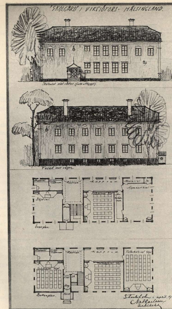
19. Förslag till skola i Viksjöfors, Hälsingland.
