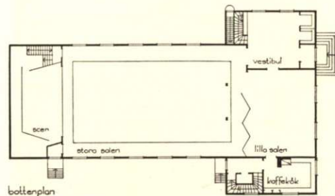
Planerna. Den vinkelställda byggnadskroppen inrymmer den stora samlingsalen.
