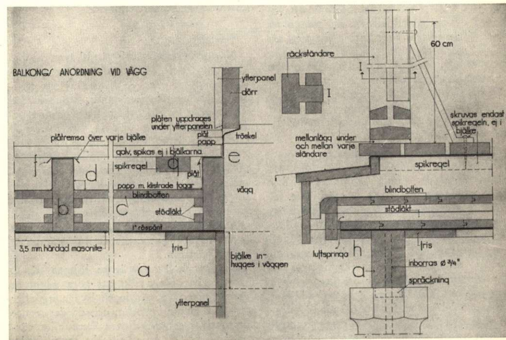
Fig. 3. Detaljritning visande konstruktionen av verandan i fig. 2.
