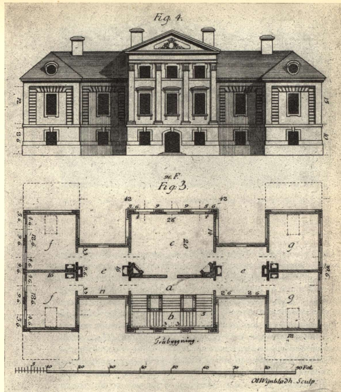
Ur Carl Wijnblads arbete »Ritningar på fyratio wåningshus af sten och trettio af träd samt åtskilliga lusthus» — 1700-talets typritningar.
