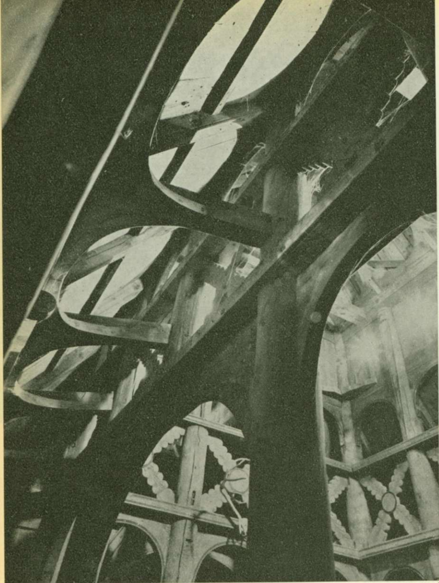
Norsk stavkyrka från 1100-talet. Borgund i Sogn. — Våldiga mastresningar stå på en enda sylldram. De styras och hållas i läge medelst ett invecklat system av bomlag, kryssförsträvningar och självvuxna gren eller rotklykor. De sistnämnda är ett ålderdomligare moment än bommar och kryss, besläktat med urgammalt båtbyggeri.
