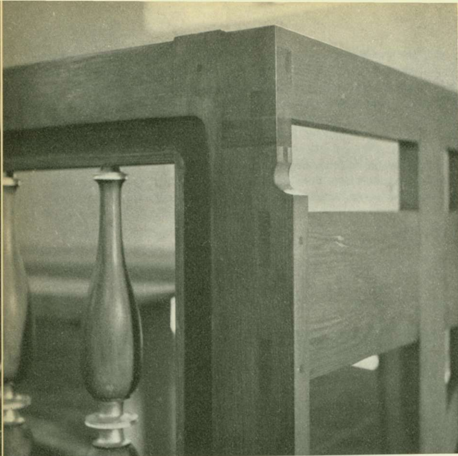
Bänkskärm i Skällviks kyrka, Östergötland. — När vi fogar samman en träkonstruktion — utan metallers hjälp — gäller det att åstadkomma god fasthet och att foga så att inte virkets krympning och svällning förstör fogningen. På bredden rör sig virket ganska mycket allt efter årstid, värme, fuktighet. På längden finns praktiskt taget ingen rörelse alls. Svårast att klara är därvid sammanfogningen av tre virken i en och samma knutpunkt.
