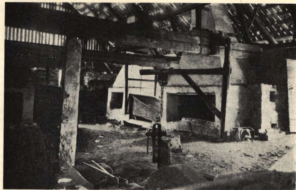
Fig. 8. Interiör av klingsmedjan vid Wira bruk, Uppland. (Efter restaureringen.)
