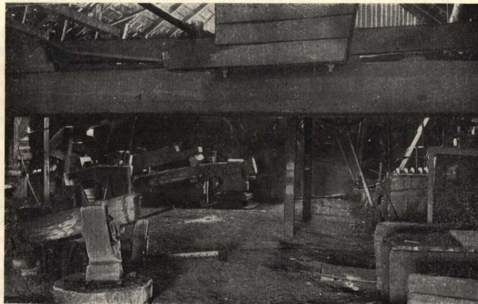
Fig. 7. Interiör från Häfla övre hammarsmedja, Östergötland.
