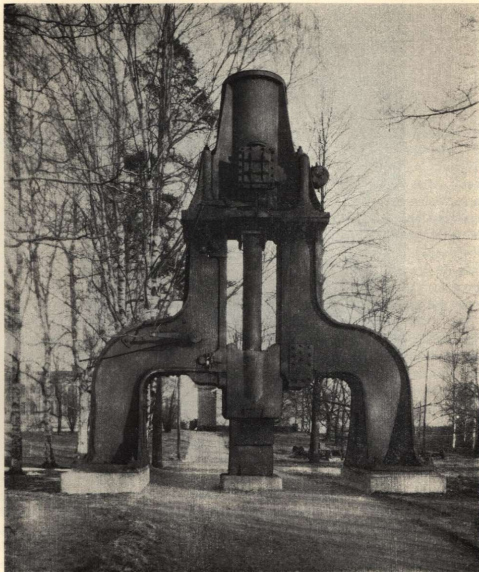
Fig. 2. Ett av vårt lands främsta tekniska minnesmärken. — 15 tons ånghammare från år 1863 använd vid Sandvikens Jernverks A.-B. År 1933 uppställd i parken vid verkstäderna som ett minnesmärke.
