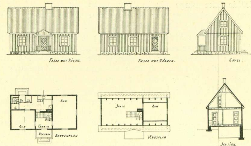
Förslag till boningshus för en familj i Tjörnarps (norra Skåne). Skala 1/400. Utfört vid Byggmästareskolan på Heltan 1927.
