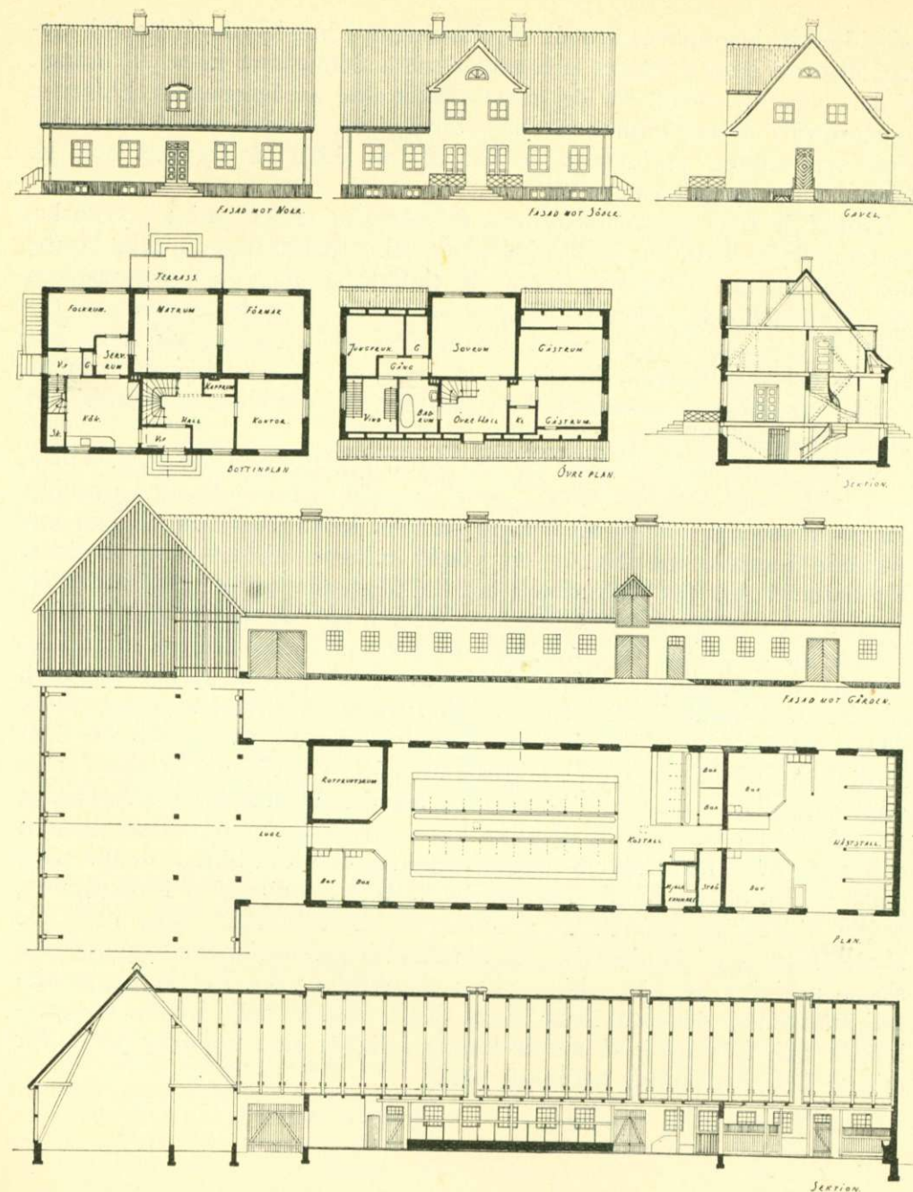
Förslag till boningshus och ekonomibyggnader för 90 tunnlands jordbruk på skånska slätten. Skala 1/400. Utfört vid Byggmästareskolan på Heilan 1927.
