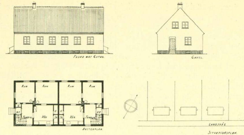
Förslag till stathus för två familjer (skånska slättbygden). Skala 1/400.
