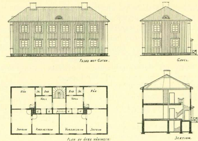
Förslag till bostadshus för fyra familjer i ett småländskt samhälle. Skala 1/400.
