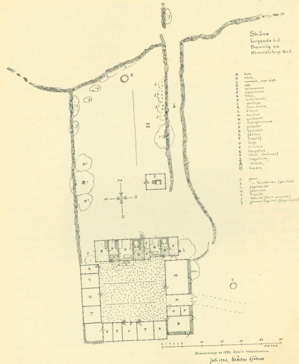
Plan av Himmelstorp n:r 1, Brunnby s:n. A kök, B »stua», C kammare, D kök, E spiskammare, F pigkammare, G stua, H »lilla hused», I förstuga, K »stora hused», L »bihave», M kostall, N »gadeport», O drängkammare, P fölkätte, R häststall, S fårhus, T loggolv, U loge, V svinhus, X hugghus, Y »sters» (förr bränneri), Z »blegebacke», Å »sträde», Ö brunn, a päron, b »bunketiner», c fågelkörsbär, d plommon, e humle, f rödvilde (Salix purpurea), g gammal liguster. Delvis rekonstruerad med hänsyn till planens utseende c:a 1880. Uppmätning av författaren.
