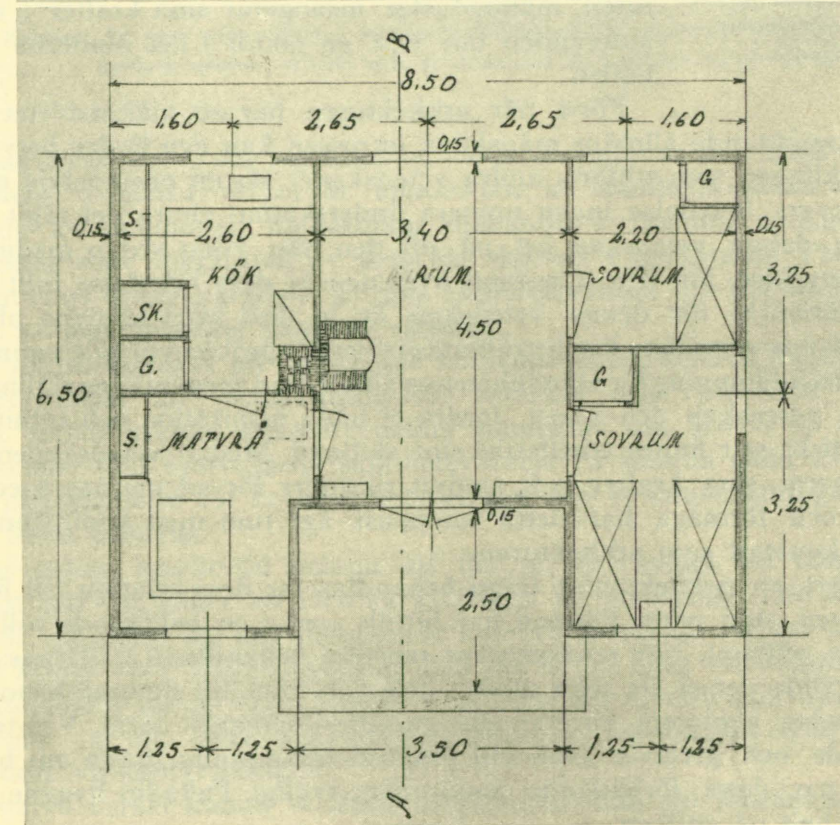
Förslag till sommarstuga upprättat på byggmästarens skola. å Hvilan.
