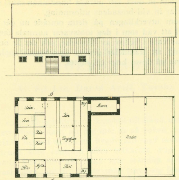
Typritning till småbruk i norra Sverige. Ladugården.
