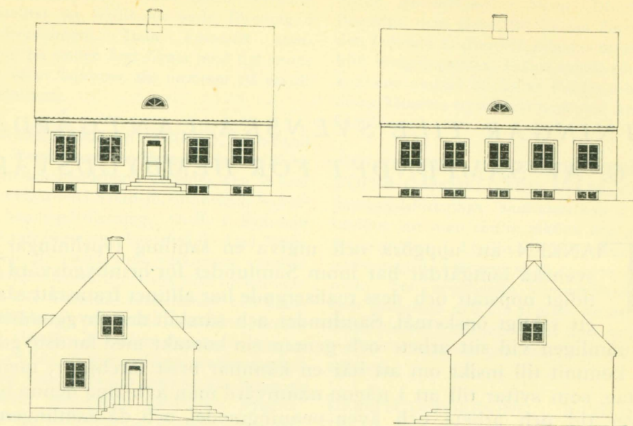
Typritning till småbruk i sydligaste Sverige. Bostaden.
