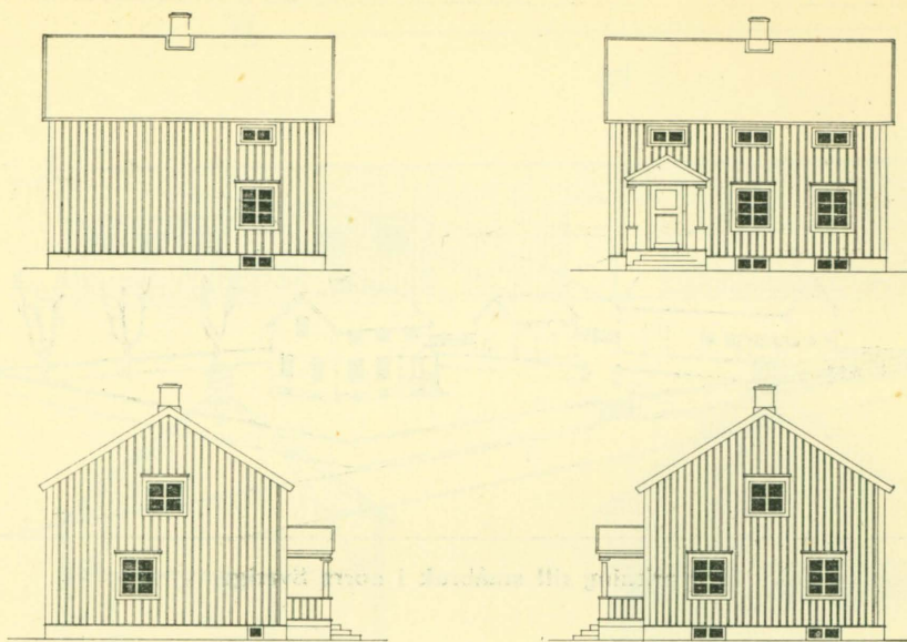
Typritning till småbruk för norra Sverige. Bostaden.
