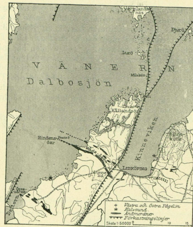
Karta, visande land- och kustformens uppkomst kring Kinnevik och Kållandsö.
