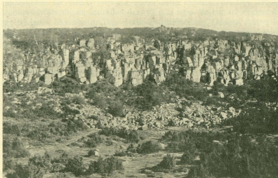
Gammal lavabädd, diabasväggen i Gerumsberget på Falan.
