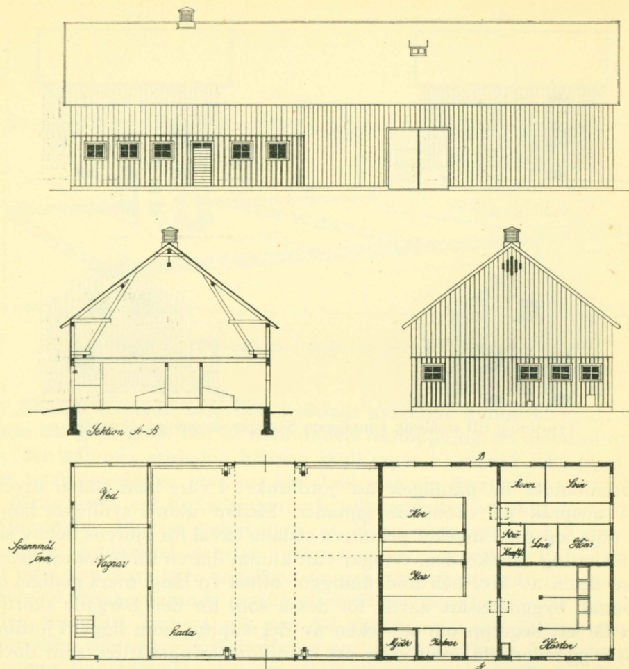
Typritning till småbruk i mellersta Sveriges skogsbygd. Ladugårdsbyggnaden.
