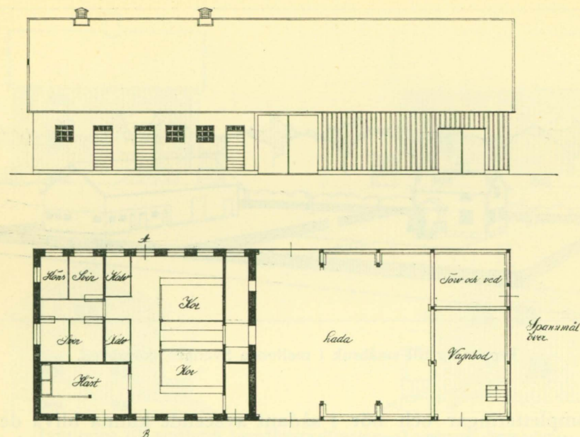
Typritning till småbruk för sydligaste Sverige. Ladugårdsbyggnaden.
