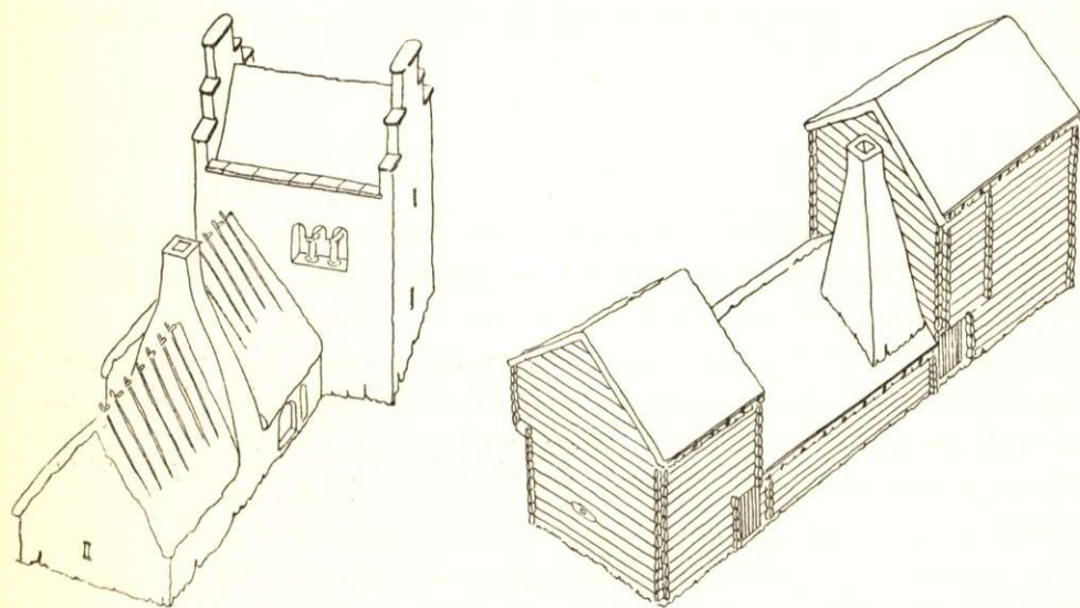
Fig. 24. Medeltida prästgård i Lau, nu bevarad blott såsom ruin. Bilden försöker rekonstruera dagligstugan, som har haft spisel och bakugn bredvid ingångsdörren. Både spisel och rummets ingångsparti har legat under en stor kupolartad rökhu. Denna har vilat på en valvbåge, spänd tvärs över rummet. — Fig. 25. Spiseln i Kyrkhultstugan på Skansen. Här i ett timrat hus har man inte kunnat bygga valv och kupolhu utan spiseln bär sin skorsten själv. Bakugnen har dessutom fått sin egen hård, skild från hörnets större spisel. — 26. Lau prästgård sedd utifrån. Försök till rekonstruktion. Gårdens boningshus har bestått av en murad loftbod och en därmed sammanbyggd stuga. — Fig. 27. Kyrkhultstugans baksida med den mäktiga skorstenen. Jämför fig. 26.
