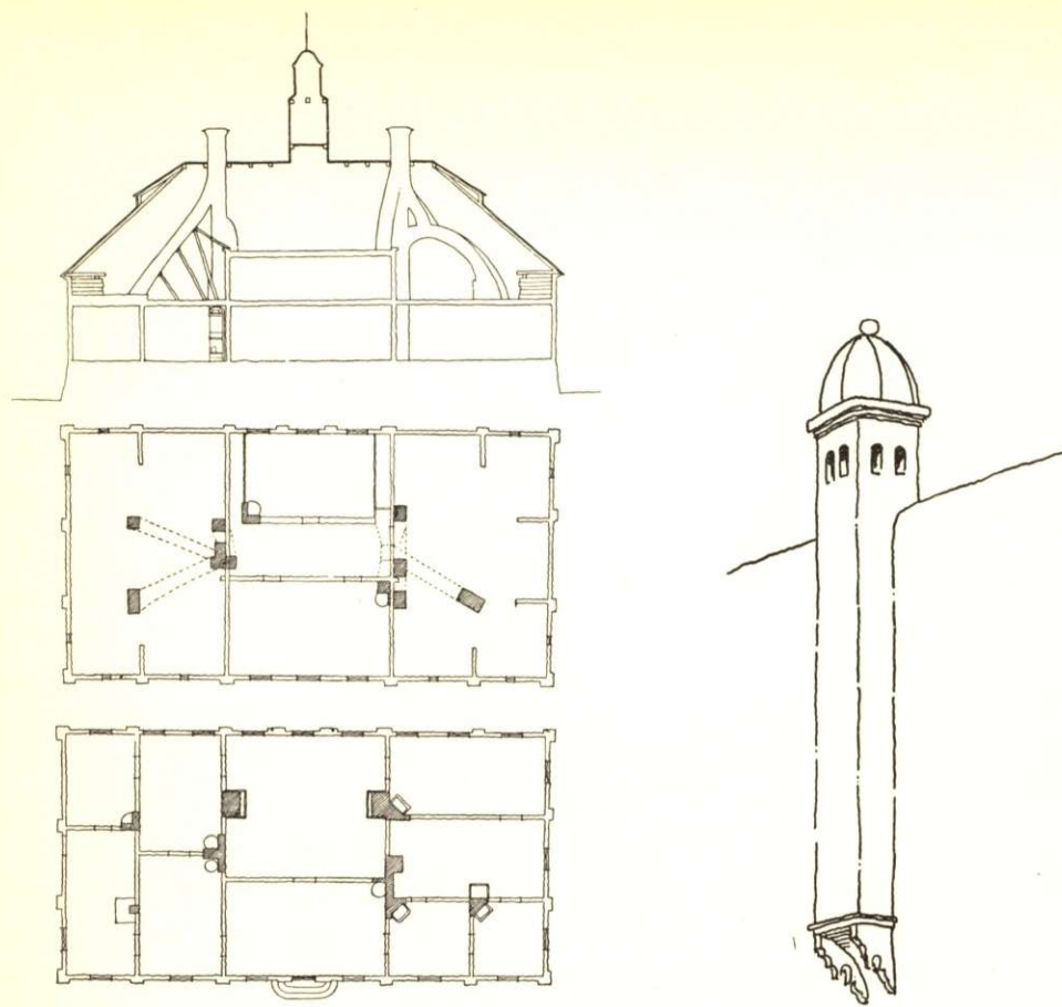
Fig. 5. Svensk timrad herregård med rumsguppering i dubbla filer. Rökrören knippas ihop till tvenne skorstenar i taknockens linje. — Fig. 6. Utbyggd skorsten, Marocko.
