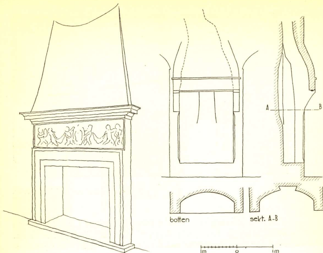
Fig. 9. Italiensk spisel med eldstad av låg typ. — Fig. 10. Spisel från 1530-talet. Malmöhus slott i Malmö. Spiselns öppning är manshög. I ryggen en urtagning, som avsågs befordra draget.
