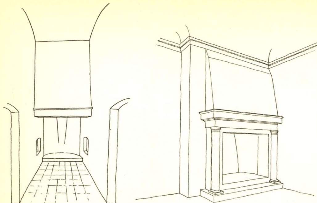
Fig. 17. Spiseln fig. 13 i rekonstruerat skick. Den står i ståthållarevåningens förstuga på Malmöhus och har tjänat för matlagning i viss utsträckning. Från spiseln ha de omgivande rummens biläggargugnar eldats. — Fig. 18 Svensk eldstad av typ liknande fig. 9. Från Östermalma i Södermanland.
