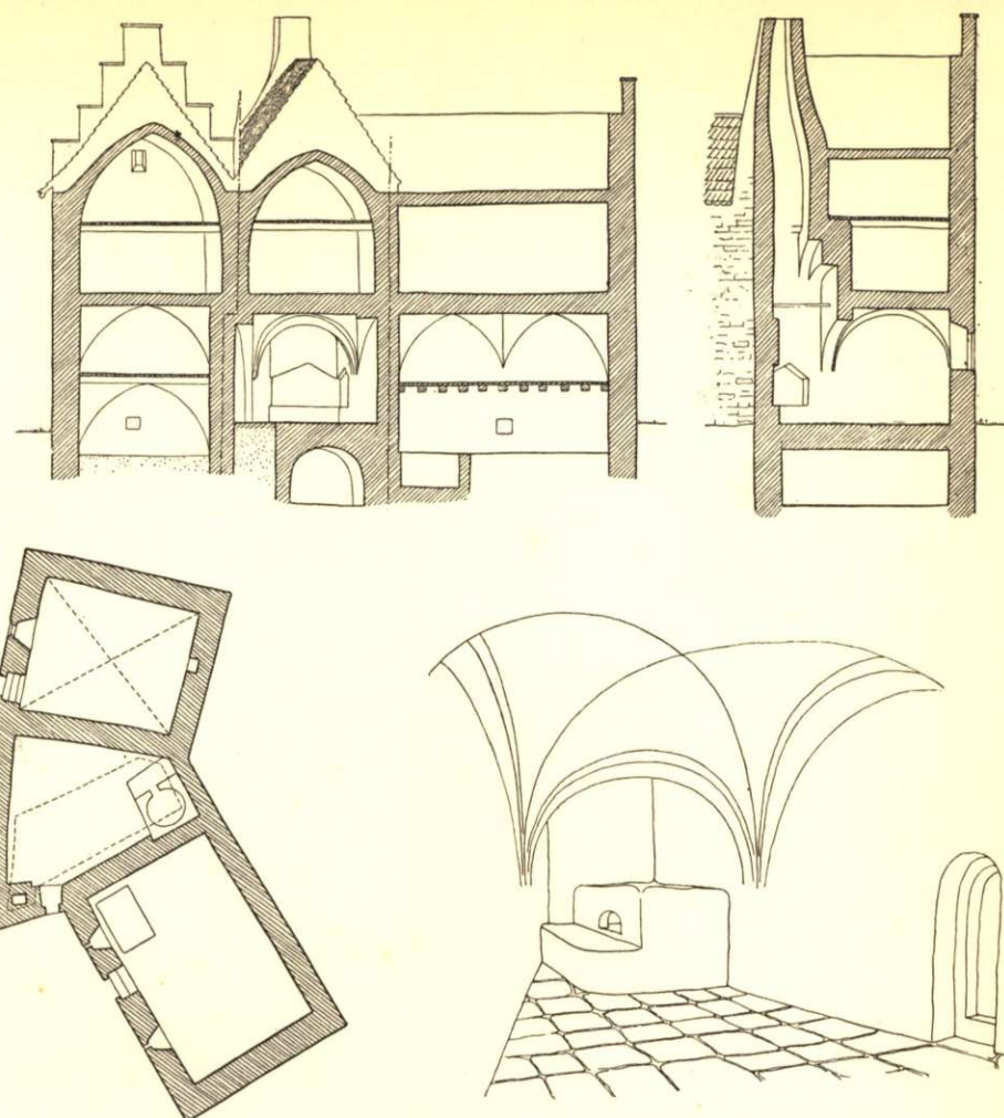
Fig. 31. En visbyköpmans dagligstuga på 1300-talet. Från Häggska huset i Visby. Profil, plan och perspektiv. Rummet täcktes av ett kryssvalv; en god del av rummet upptages dock av en väldig rökhuv med skorsten. Under huven har bakugn och hård varit anbragta.
