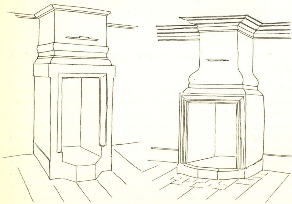
Fig. 19. Karolinska spisar i timmerhus (Sveden, Dalarna). Hela rökgången vilar på spisels murkub. Omfattningen kring härdens öppning är i sådana spisar ofta av huggen sten, men ej sällan är den murad av tegel samt putsad. Det förekommer också att profilen är gjord i trä och lagd såsom ett vanligt foder kring öppningen.
