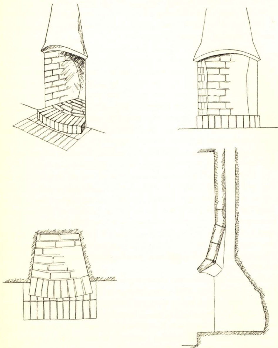
Fig. 32. Modern spisel med uppsvängd kupa. Kupans välvda kant bär sig själv utan järnunderlag. Den belastas och hålles i läge genom huvens övre delar.
