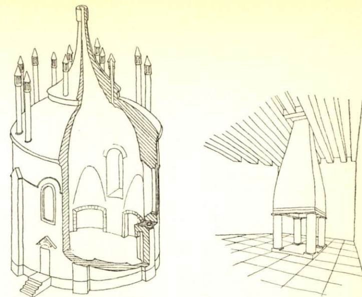
Fig. 20. Ett franskt klosterkök från medeltiden. Byggnaden är egentligen en rökstuga i jätteformat. Taket har en rököppning i mitten och utgör en rökhu, som spänner över hela det runda rummet. I detta fall är en hel rad spisar murade invid ytterväggarna. De ha sina egna skorstenar. I dessa spisar lagas maten över öppen eld. — Fig. 21. Slottskök från 1500-talet. Stekspiseln i rummets mitt omges av fyra stenpelare, som bära upp rökhu och skorsten. Här stekas oxarna hela, upprädda på spett. Denna sort av kök motsvarar fig. 20 och 22, fastän rökhuven inte omfattar hela rummet utan blott själva härdens.
