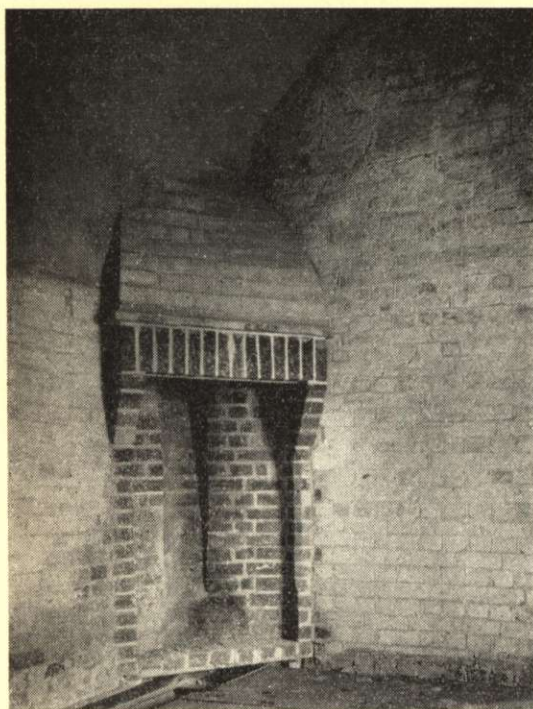
Fig. 12. Hörnspisel på Malmöhus. — Fig. 13. Bild av spisel på Malmöhus, tagen före rekonstruktionen av huven. Man ser här hur urtagningen i ryggen är anordnad.
