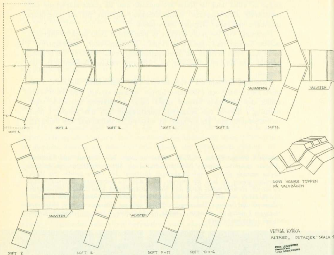
Altaret i Veinge. Konstruktionsritning som anger tegelstenarnas läge skift för skift. Det har här gällt att ge stenförbandet just det åsyftade sammanhanget, segheten i murningen. Först genom dylikt studium av stenarnas inbördes förhållanden vinnes den arkitektoniska formen.
