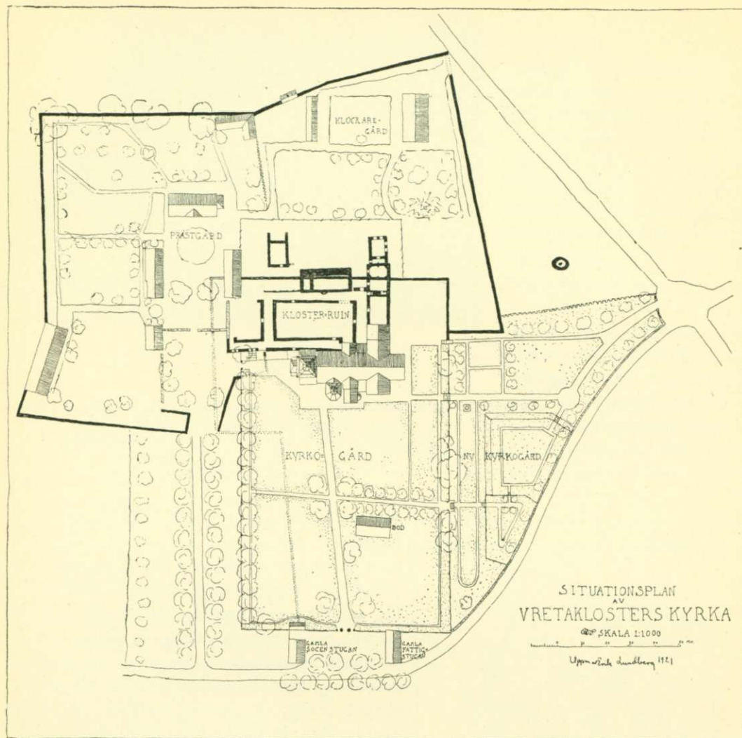
Situationsplan av Vretakloster med kyrkan och prästgården. Uppmätning för "Sveriges Kyrkor" av Erik Lundberg 1921.
