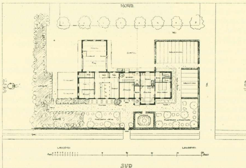
Förslag till mindre lantgård på Jylland. Fasad och plan. Arkitekt: H. Kampmann.
