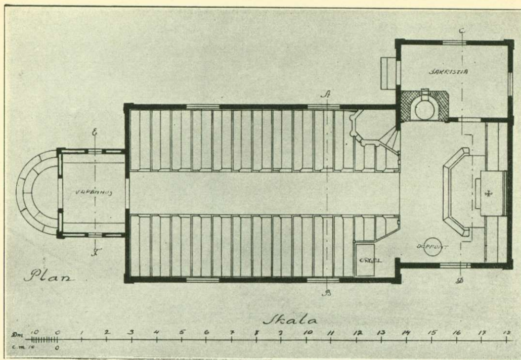
Slädene kapell. Arkitekt: Knut Nordenskjöld. Plan.
