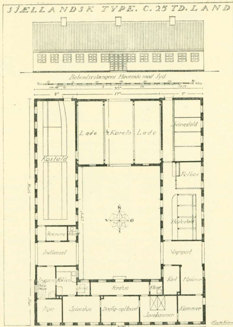
Förslag till själländsk gård om c:a 25 tunnland. Fasad och plan. Ur "Danske Landbrugbygninger".
