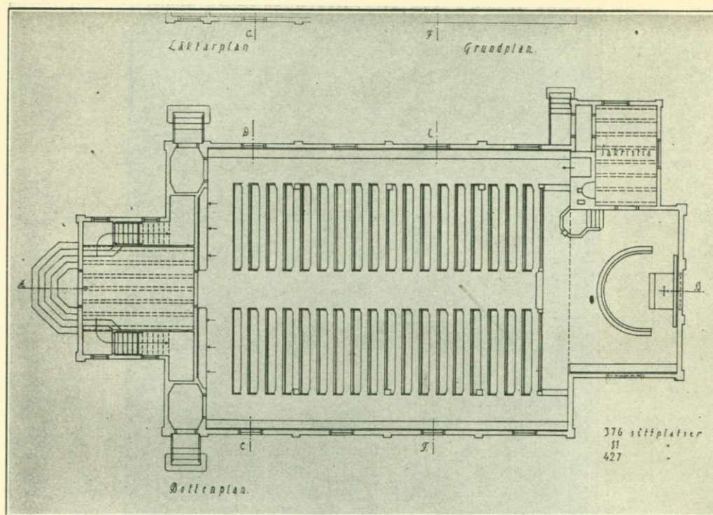
Norrfors kyrka. Arkitekt: Knut Nordenskjöld. Plan.
