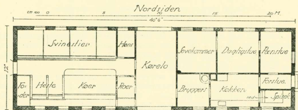
Förslag till själländsk gård om c:a 8 tunnland. Ur "Danske Landbrugsbygninger".
