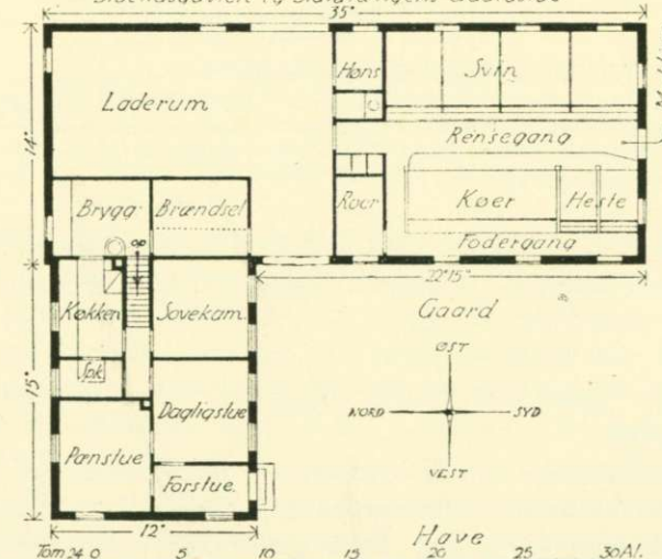
Förslag till jylländsk gård om c:a 12 tunnland. Fasader och plan. Förslag utarbetat av "Bedre Byggeskikks Tegnehjælp".
