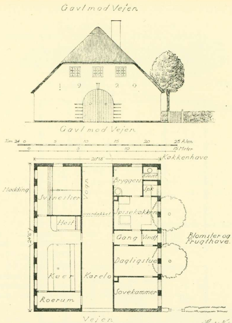
Förslag till jylländsk gård om c:a 8 tunnland. Ur "Danske Landbrugsbygninger" *).
