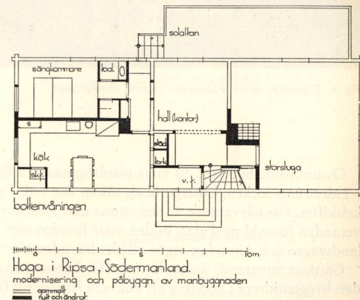
Fig. 6. Förslag II, plan av bottenvåningen.
