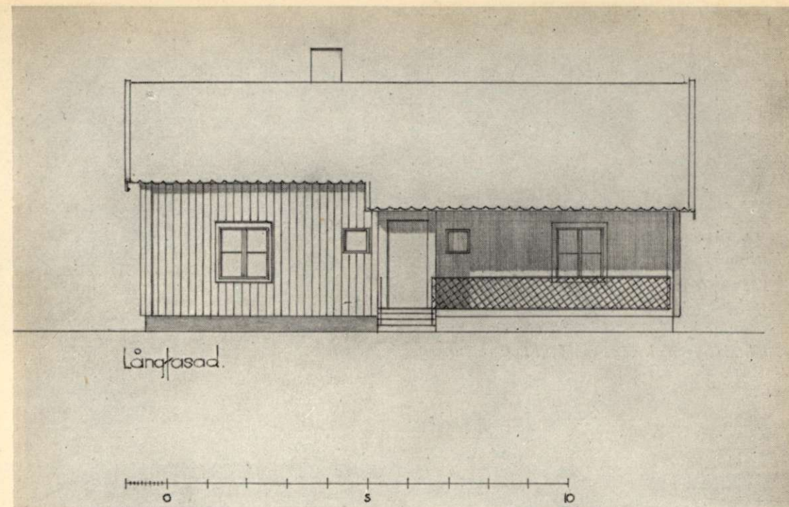
Fig. 12. Den gamla parstugan låter sig med fördel modernisera. Här ett förslag.
