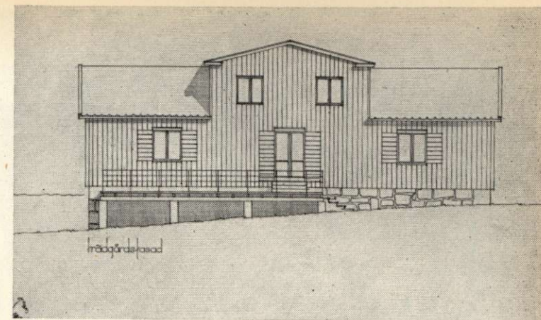
Fig. 5. Förslag II till modernisering av Haga gård; trädgårdsfasad.
