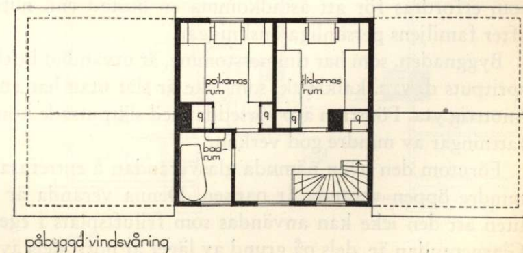
Fig. 7. Förslag II, plan av påbyggd vindsvåning.
