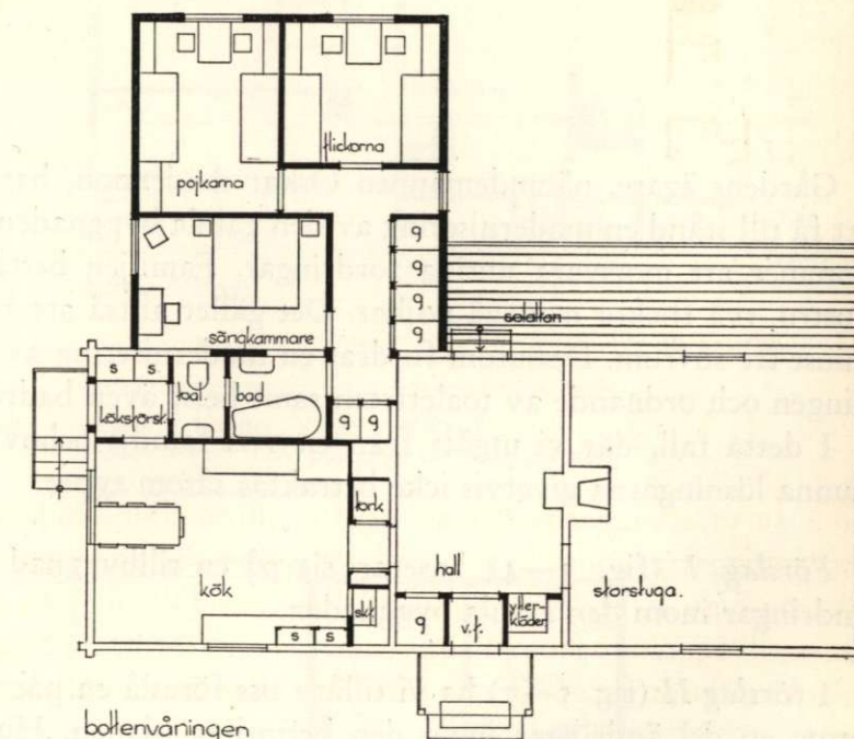
Haga i Ripsa, Södermanland modernisering och tillbyggn. av manbyggnaden. — gammalt — nytt och ändrat
