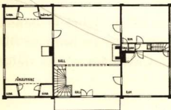
PLAN AV VÅNINGEN 1 TR.
