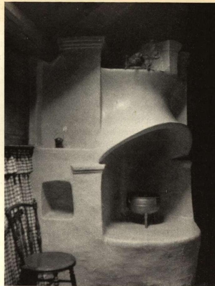
Den öppna spisens valv, Lustorp, Köinge.
