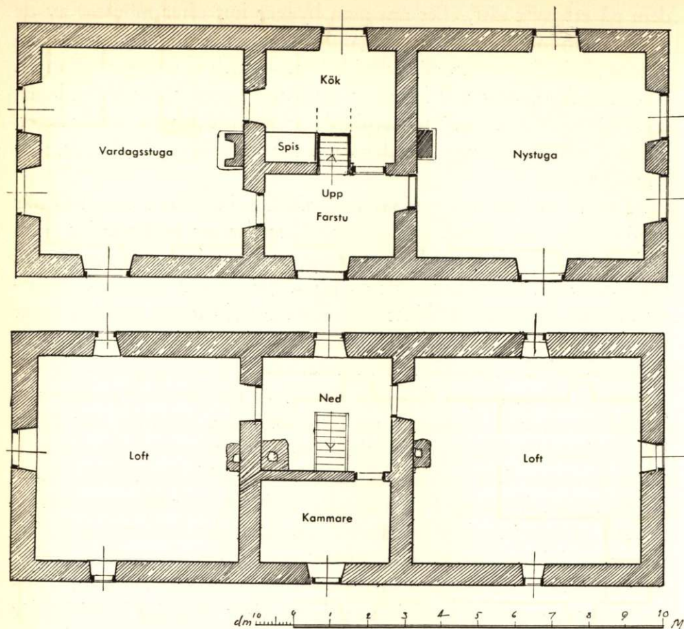
Fig. 4. Plan av en gammal gottländsk parstuga.
