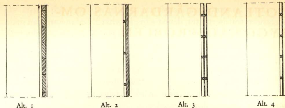
Fig. 1. Olika konstruktioner för erhållandet av täta ytterväggar: Alt. 1. Kalkstensmur 4 cm. lufttrum, 8 cm. plåtar, innerst puts. Alt. 2. Kalkstensmur 1\frac{1}{2}'' \times 1\frac{1}{2}'' regler på 60 cm. avstånd, 3 cm. träullsplatta, innerst puts. Alt. 3. Kalkstensmur 1\frac{1}{2}'' \times 1\frac{1}{2}'' regler på 40 cm. avstånd, 12 mm. porös träfiberplatta. Alt. 4. Kalkstensmur 1\frac{1}{2}'' \times 1\frac{1}{2}'' regler på 40 cm. avstånd, 6 mm. halvhård träfiberplatta. Alt. 5. Kalkstensmur 1\frac{1}{2}'' \times 1\frac{1}{2}'' regler på 40 cm. avstånd, 12 mm. porös träfiberplatta.
