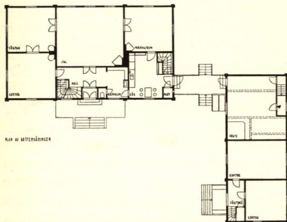
Plan av bottenvåningen.
