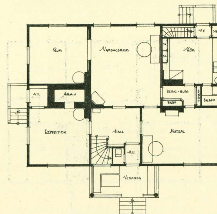
Bottenplan. Silleruds prästgård.
