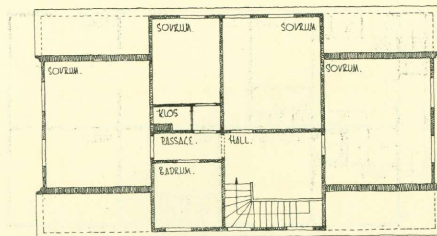
Plan 1 trappa upp. Adolfsfors prästgård.
