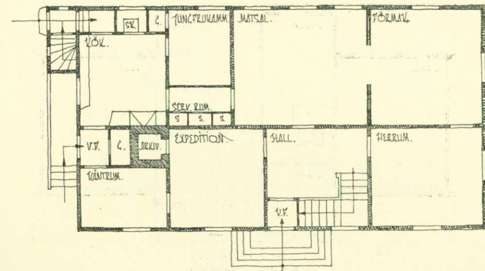
Bottenplan Adolfsfors prästgård
