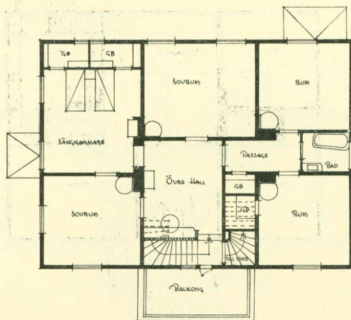
Plan 1 trappa upp. Silleruds prästgård.
