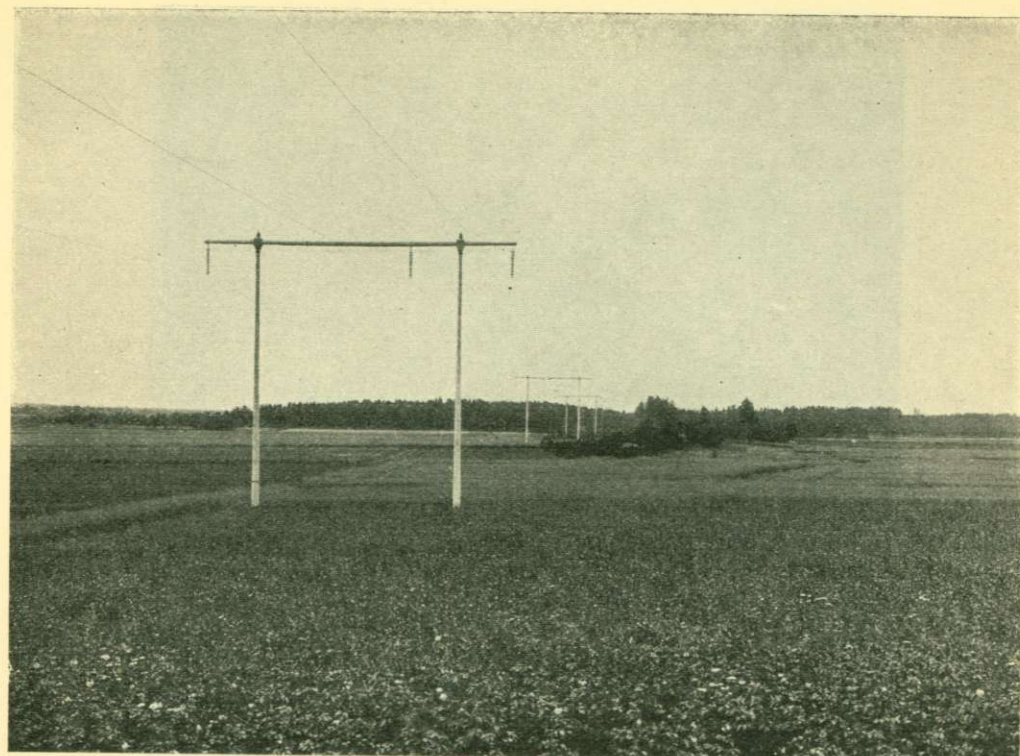
Kraftledning med stolpar av betong. Kungl. Vattenfallsstyrelsen.
