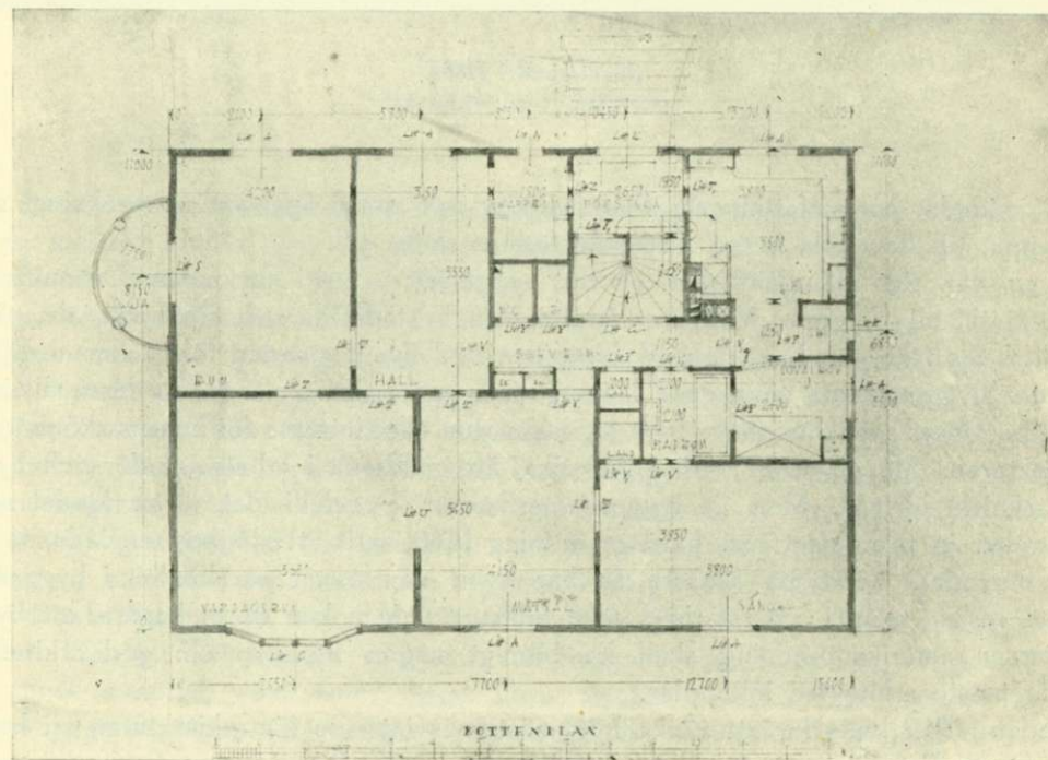
Bostadshus i Östersund. Stadsarkitekt I. Stål, Östersund.
