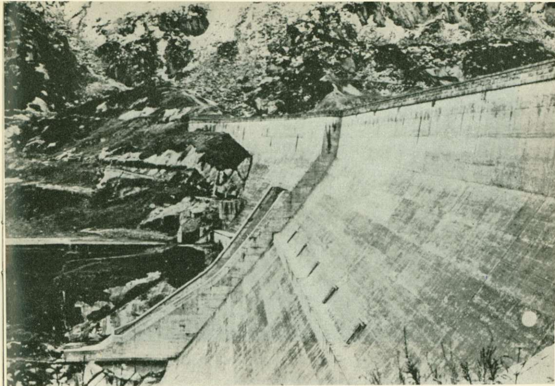
Den stora betongdammen i övre Hassli i Schweiz. — Foto: J. Nihlén.
