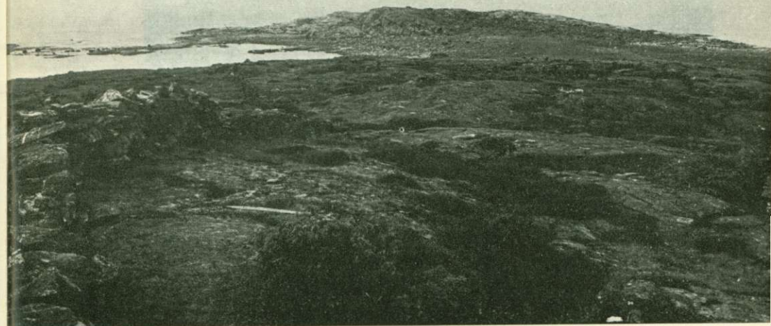
Den vackra Ringhalsudden med sina fårbetade marker, vindformade enar och ljung blir ett säreget naturreservat i skuggan av det stora atomkraftverket. – Foto T. Nihlén.
