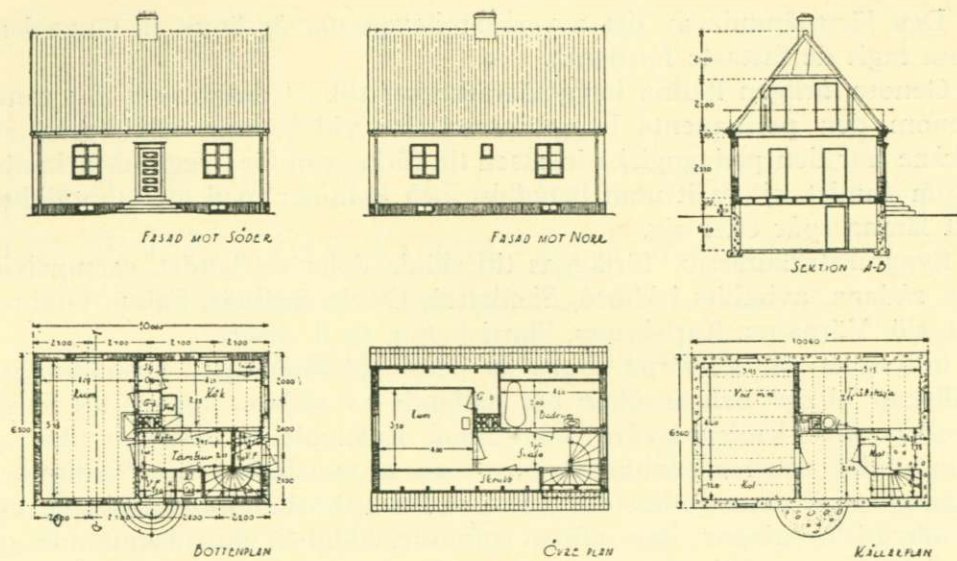
Förslag till arbetarbostad för en familj. Samfundets byggmästareskola i Åkarp 1929.
