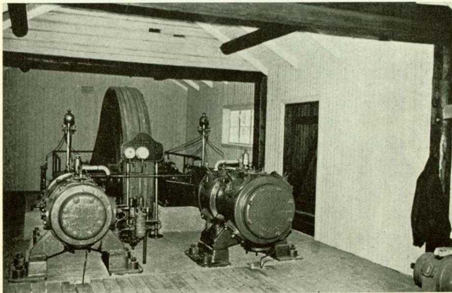
Senaste utökningen på Gruvmuseet är Atlas-huset, som innehåller en kompressor av äldre modell, avsedd att gå i sakta fart, driven av en el-motor på ett par hundra hästkrafter.
