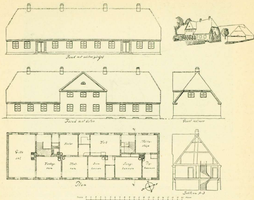
Förslag till boningslänga på skånsk lantgård, utförd på folkhögskollärarkursen 1918.
