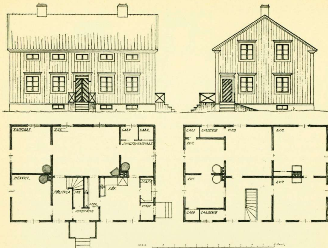
Förslag till manbyggnad på jämtländsk gård, utförd vid byggmästarekursen i Östersund 1919.
