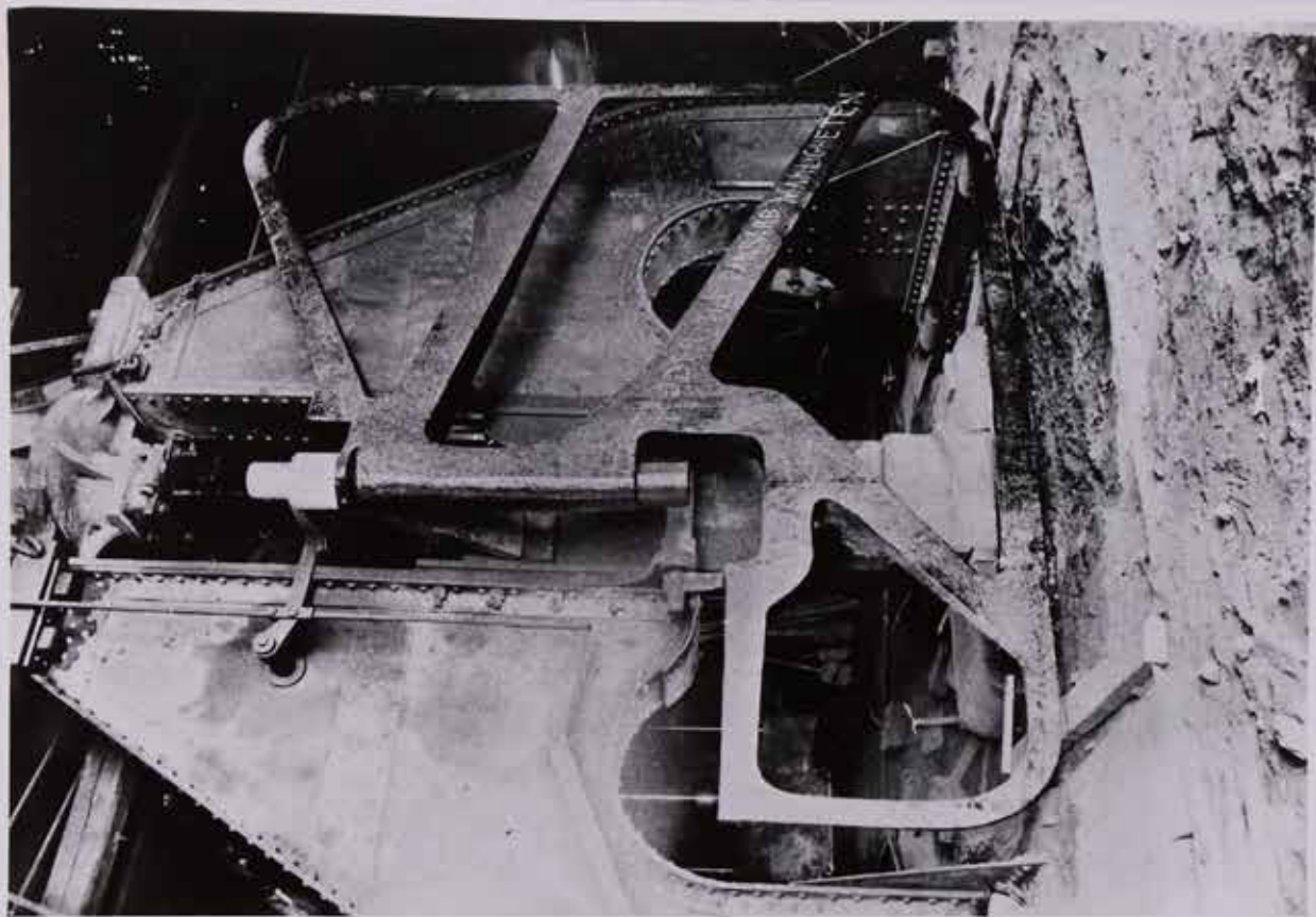
LOTORPS ENGELSKA ANGHAMMARE -Brukets stolthet- Sades vara Europas största, när den var i arbete skakade hela Bruksområdet. Foto 1905. Se även vidstående bilaga. I arbete är ett roder till pansarbåten "Manligheten". Anghammaren hitkom 1897, effekt 10 ton. Nedmonterad 1919 och förd till Kolsva där den var i bruk till 1954.
