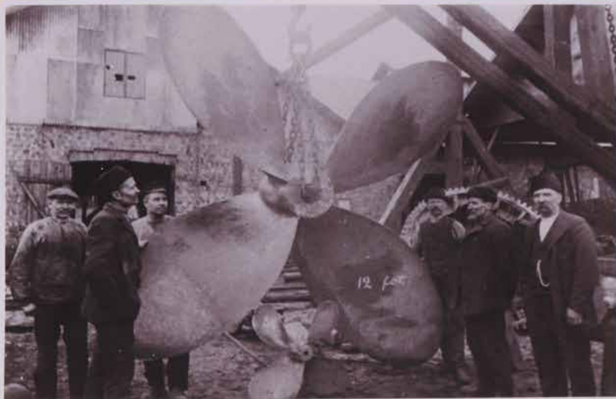
Maskindelar till pansarbåten "Manligheten" tillverkade vid Lotorps Bruk. Övre bild märkt: "axelbärare till Manligheten vikt 1,900 kg". Nedre bild taget utanför gjuteriet fartygspropeller till Manligheten, märkt "12 fot" (=3,56 meter) Manligheten började byggas 1901, och sjösattes 1903. Var 15 meter bred och 89,7 meter lång, var i bruk till år 1950 då betydligt omändrad och moderniserad. Se även sid.6 upp.
