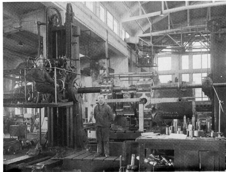
Stora arborrverket 1936. Arborraren är Ernst Ståhl och lärlingen på manöverbryggan Runo Lindvall. Arbetsobjektet är ett s k legoarbeta, en hydraulisk press till Liljeholmens kabelfabrik. Vikten på huvudkomponenten är 14 580 ton.
