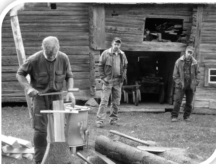
Spingning: Byggnadssnickare Börje Samuelsson tillverkar takspån, eller takstickor, vid Smedstorps dubbelgård i augusti. Foto: Bengt Björner
