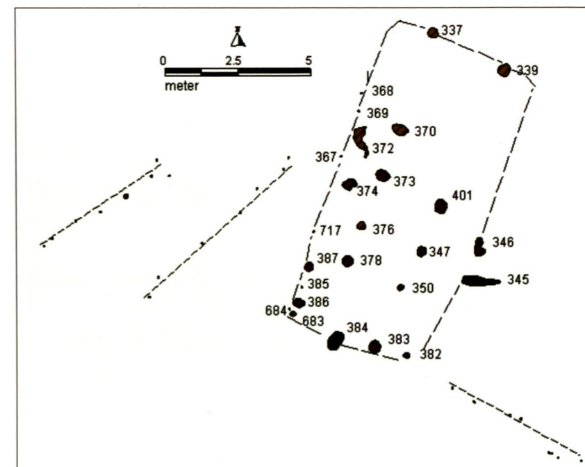
Bilden föreställer ett plan av ett treskeppigt hus från förromersk järnålder vid Tuna kyrka i Medelpad.
