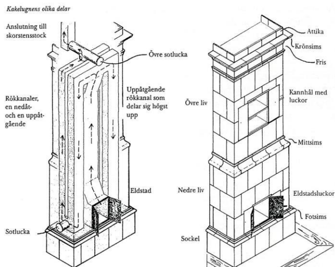
Kakelugns olika delar. Ur planschen Kakelugnar.
