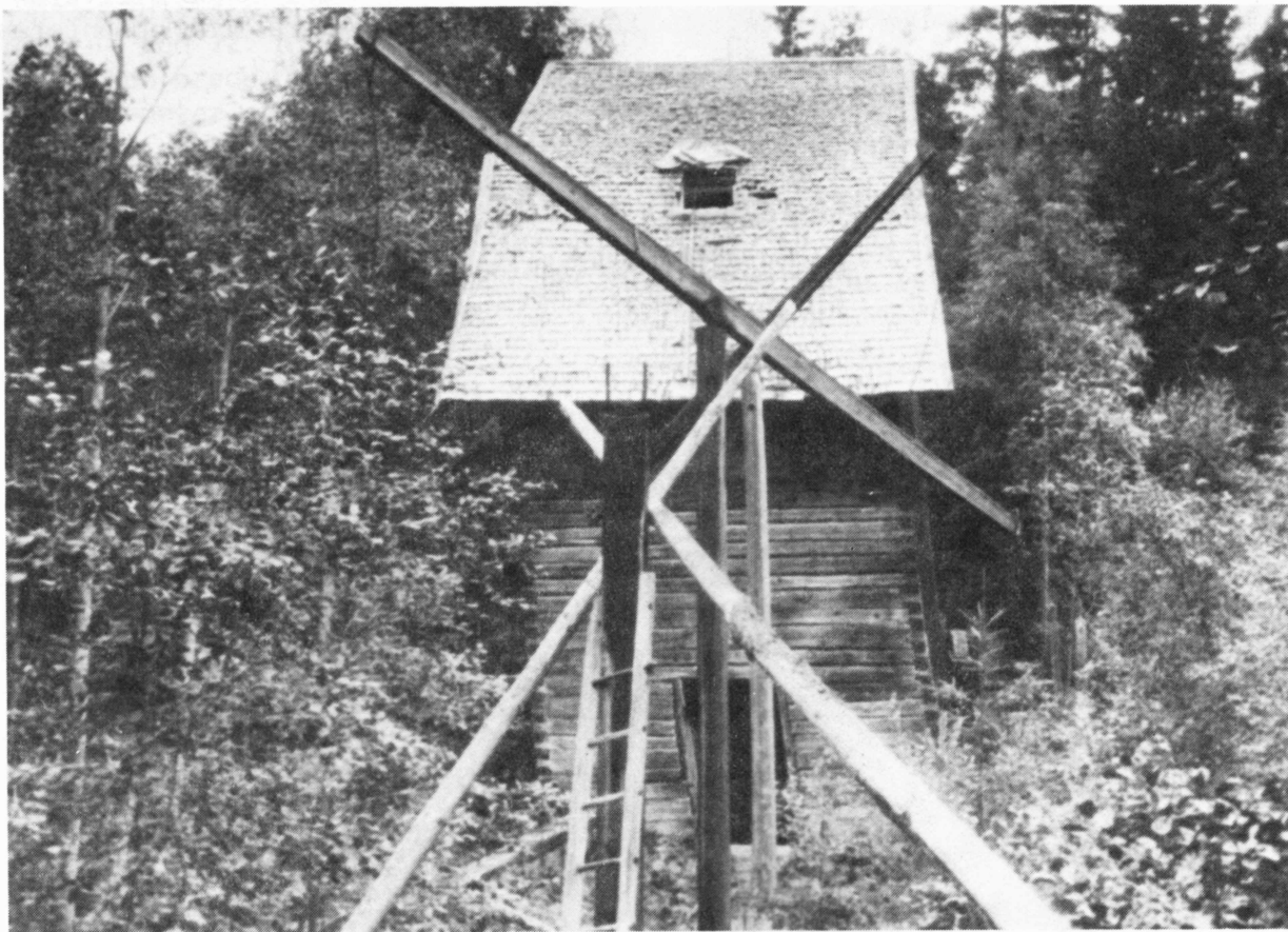
Bild 7. Östanbergshjulets hjulhus med början av stånggången.
