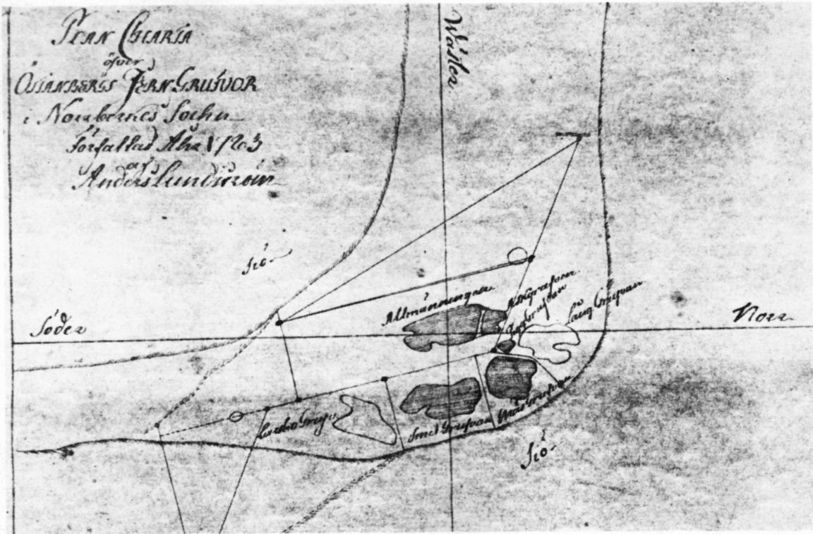
Bild 4. Gruvkarta från 1783.
