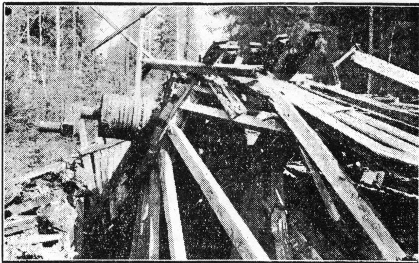
Bild 9. Det sammanstörtade hjulhuset våren 1930.
