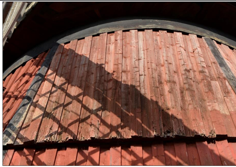
Rötskadad lockpanel på fasad mot sydost, åtgärdas 2021. Foto: AP, 20200917
