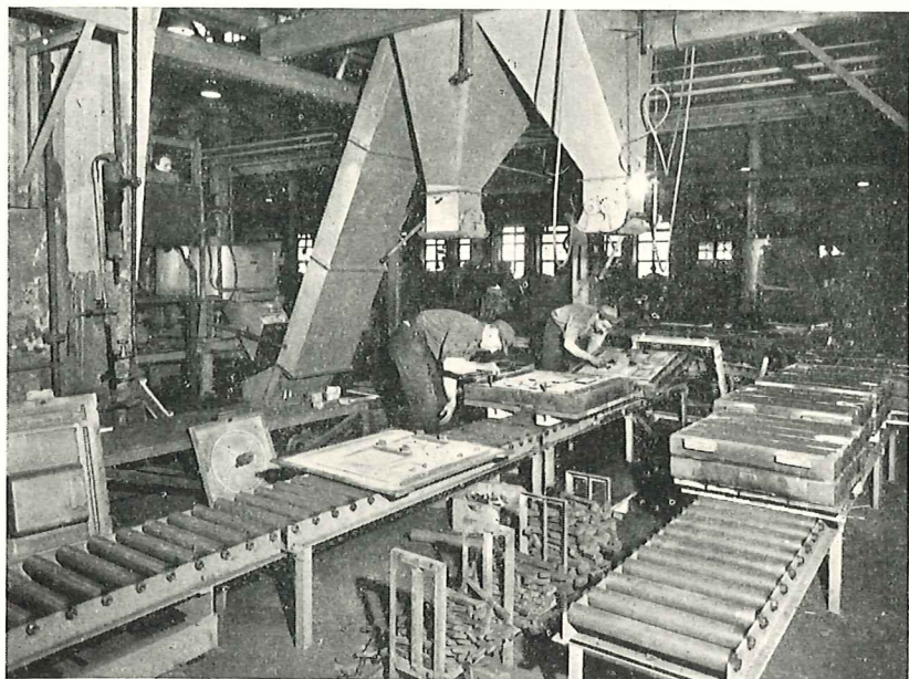
Mekaniserad formningsavdelning vid AB Pump-Separators Gjutrier.
