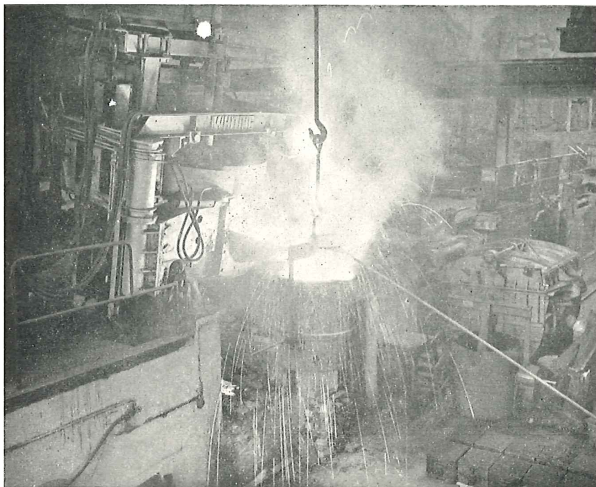
Ståltappning vid ljusbågugnen i S. K. F.
