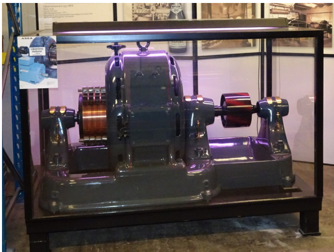
Likströmsmotor i glasmonter, märkt 30 hk, 650 HV (rpm). Motorn är renoverad och funktionsduglig. Huvudmotor med plattremsdraft ursprungligen levererad 1901 till Hamburgerbryggeriet i Stockholm.
