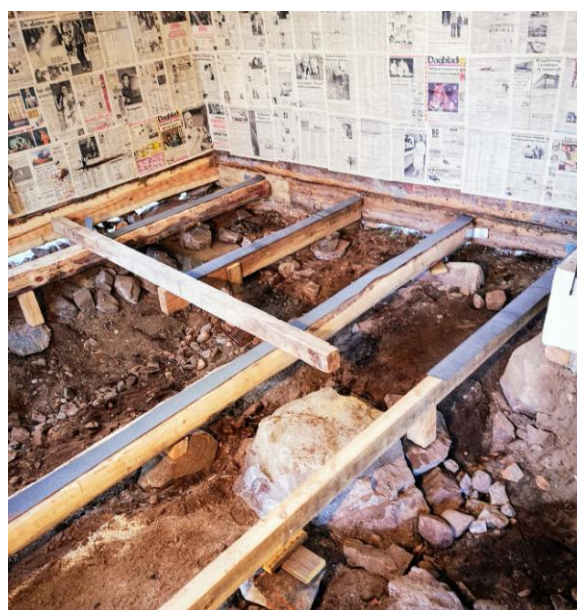
Stenen är spräckt i mindre bitar och nya golvbjälkar läggs in.
