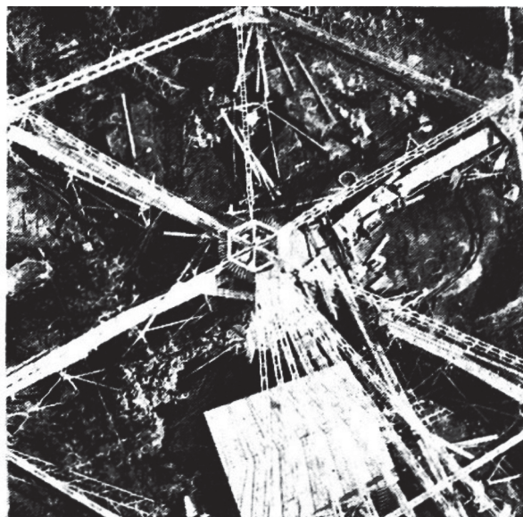
Bilden ovan visar mastmontörerna och medhjälparna. Fr. v. Ragnar Bülow, Leif Olsson, Bengt Erixon, Sten-Erik Engblom, Uno Persson och Bror Rahm. Till höger ses den 40 ton tunga reflektorn under byggnad. Bilden är tagen från toppen på en av masterna.
