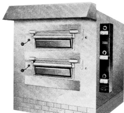
A-26 – ackumulerande platsbyggd bakugn för 6st bakplåtar i varje ugnsrums (tillv. år 1950-60)
