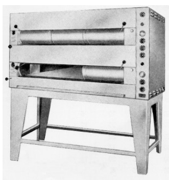
UEM 2x6 – bakugn för 6st bakplåtar i varje ugnsrums (tillv. år 1958-86)
