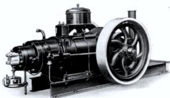
Beijer råoljemotor 25 hkr som Viktor hade i sitt sågverk
