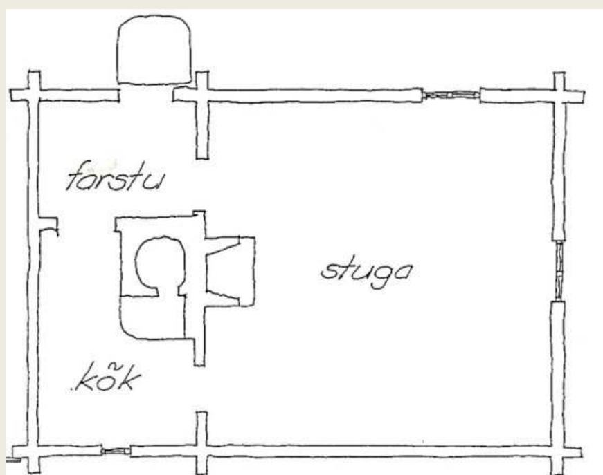
Planritning för hus i Krämarstan eller Finnerödjatorp
